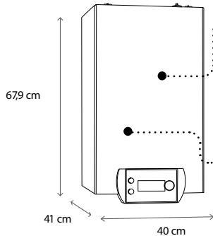
Εσωτερική μονάδα Alezio S
